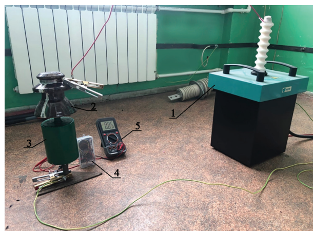
Рис. 3. Экспериментальная установка: 1 — установка АИД-70М; 2 — изолятор ШФ-10Г; 3 — высокоомный шунт; 4 — диагностическое устройство; 5 — вольтметр
