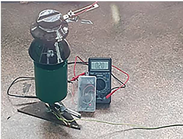
Рис. 4. Рабочее состояние диагностического устройства при поврежденном изоляторе
