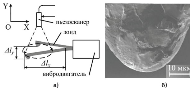
Рис. 3. Схема зондового ПАК (а) и фотография корундового наконечника (б)
