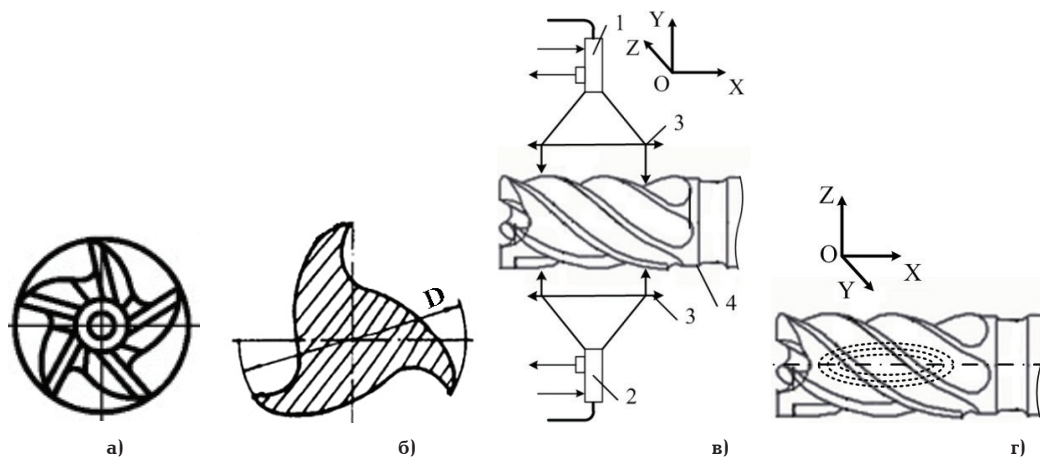
Рис. 4. Изделия с несимметричным расположением по сечению режущих кромок: фреза (а), зенкер (а) и схемы измерений размеров таких изделий: виды сбоку (в) и сверху (г)
