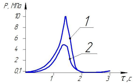
Рис. 5. График изменения давления в рабочей камере за время цикла: 1 — P_n = 10 МПа; 2 — P_n = 6 МПа Fig. 5. Graph of the pressure variation in the working chamber during the cycle: 1 — P_n = 10 МПа; 2 — P_n = 6 МПа
