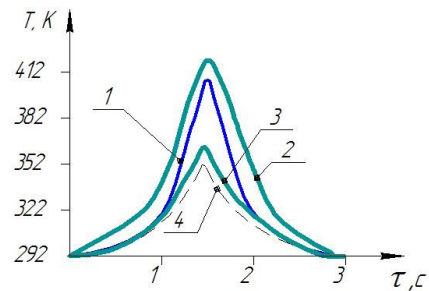
Рис. 6. График изменения температуры в рабочей камере за время цикла: 1 — режим без охлаждения, P_n = 10 МПа; 2 — режим с охлаждением ( P_n = 10 МПа); 3 — режим без охлаждения, P_n = 6 МПа; 4 — режим с охлаждением ( P_n = 6 МПа) Fig. 6. Graph of temperature change in the working chamber during the cycle: 1 — mode without cooling, P_n = 10 МПа; 2 — cooling mode ( P_n = 10 МПа); 3 — a mode without cooling, P_n = 6 МПа; 4 — a mode with cooling ( P_n = 6 МПа)
