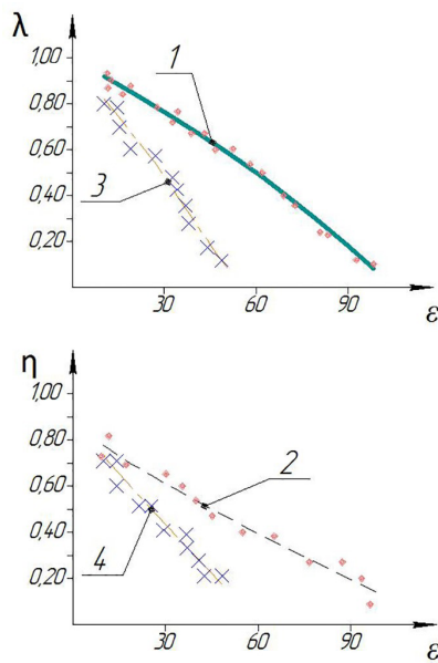
Рис. 4. Зависимость коэффициента подачи и индикаторного изотермического КПД от степени повышения давления при интенсивном внешнем охлаждении: 1 — зависимость коэффициента подачи; 2 — зависимость индикаторного изотермического КПД; 3 — зависимость коэффициента подачи при диаметре цилиндра 0,02 м и ходе поршня 0,2 м [15]; 4 — зависимость индикаторного изотермического КПД при диаметре цилиндра 0,02 м и ходе поршня 0,2 м Fig. 4. Dependence of the feed factor and indicator isothermal efficiency on the degree of pressure increase with intensive external cooling: 1 — dependence of the feed rate; 2 — dependence of indicator isothermal efficiency; 3 — dependence of the feed factor with a cylinder diameter of 0,02 m and a piston stroke of 0,2 m [15]; 4 — dependence of indicator isothermal efficiency with a cylinder diameter of 0,02 m and a piston stroke of 0,2 m
